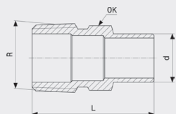
Prijelazni komad - bronca Model 94280G
