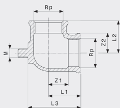
Priključno koljeno 90° Model 94477.0-713
