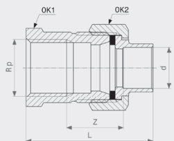
Prijelazna navojna spojnica Model 94330G
