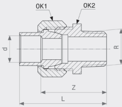
Prijelazna navojna spojnica - bronca Model 94343G
