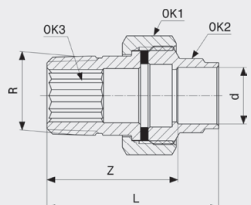
Prijelazna navojna spojnica Model 94331G
