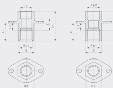
Zidna provodnica - bronca Model 3427
