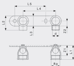
Gemini-Montažna jedinica Model 94476.21
