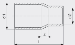
Redukcija - bakar Model 95243
