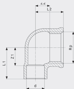
Prijelazni luk 90° - bronca Model 94090G
