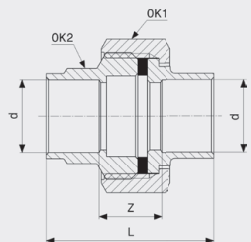
Navojna spojnica - bronca Model 94330
