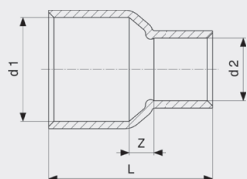
Reducir spojnica - bakar Model 95240
