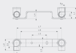
Gemini-Montažna jedinica Model 94476.0
