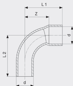
Koljeno 90° - bakar Model 95092
