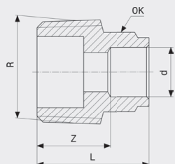
Prijelazni komad - bronca Model 94243G
