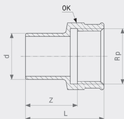
Utični komad - bronca Model 94246G
