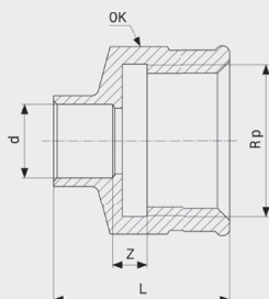
Prijelazni komad - bronca Model 94270G
