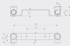
Gemini-Montažna jedinica Model 94476.1
