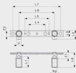
Gemini-Montažna jedinica Model 94476
