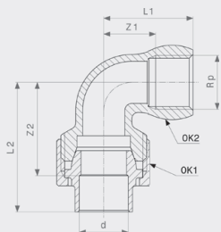
Prijelazna navojna spojnica 90° Model 94096G
