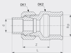
Prijelazna navojna spojnica Model 94340G
