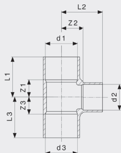
T-komad - bakar Model 95130
