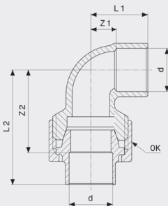
Prijelazna navojna spojnica 90° - bronca Model 94096
