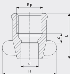
Prijelazni komad - bronca Model 94270GF
