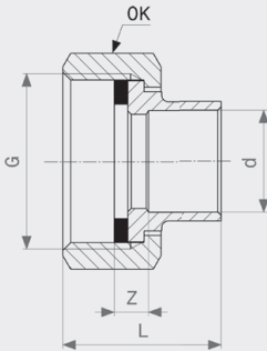
Navojna spojnica Model 94359
