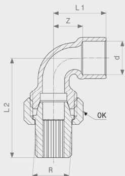
Prijelazna navojna spojnica 90° Model 94098G
