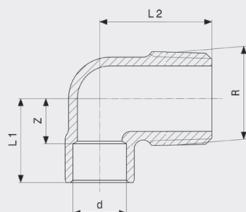
Prijelazni luk 90° - bronca Model 94092G
