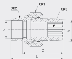
Prijelazna navojna spojnica Model 94341G
