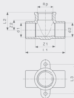
Zidna pločica sa T-komodom - bronca Model 94490G
