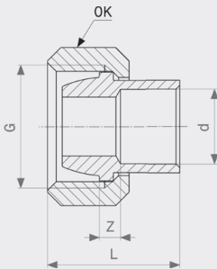
Navojna spojnica - bronca Model 94384G
