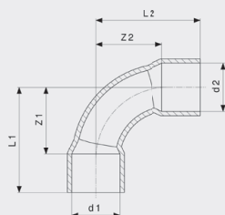
Koljeno 90° - bakar Model 95090
