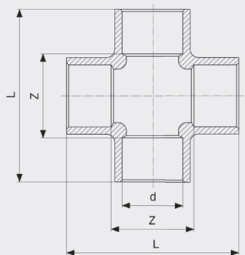
Križni komad - bronca Model 94180
